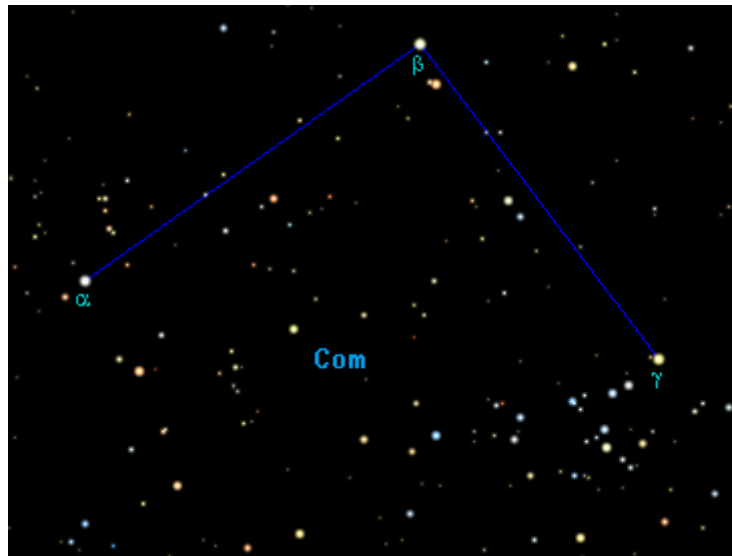
fig. 6 – la costellazione della Chioma di Berenice
