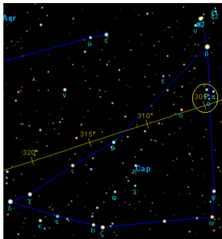
fig. 7 – la costellazione del Capricorno
