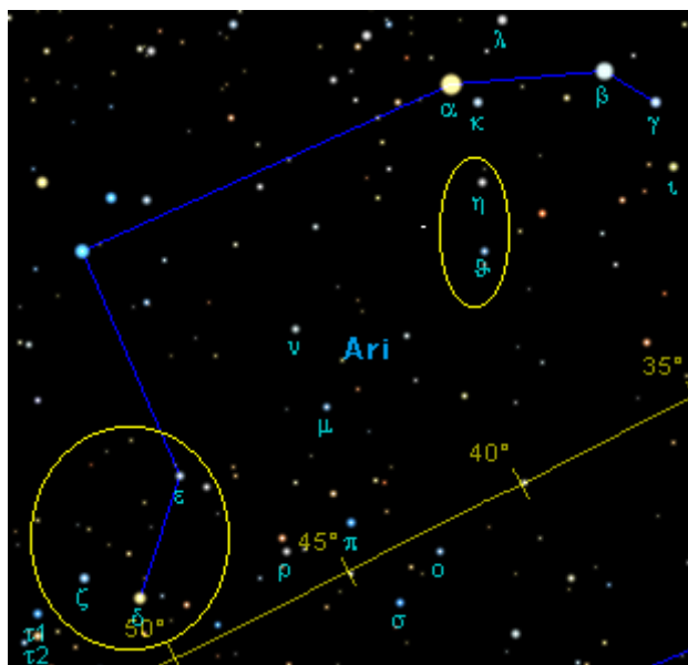
fig. 3 – la costellazione dell'Ariete
